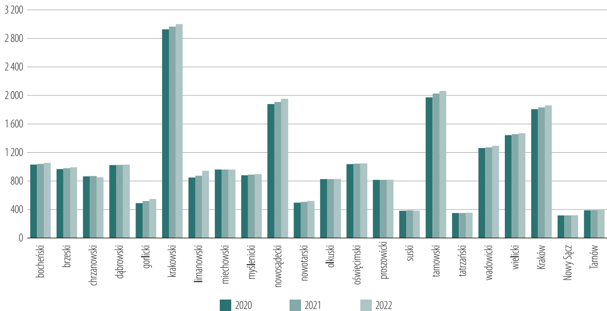
Wykres 133. Długość sieci wodociągowej w województwie małopolskim (w km)
