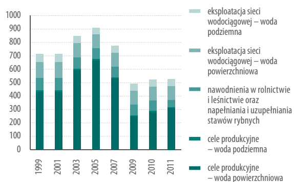
Wykres 1. Pobór wody (w hm 3 )
